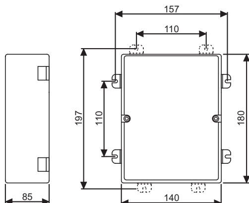
Fig.1 - DIMENSIONI (mm):
