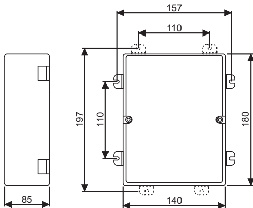
Abbildung 1 - ABMAßE (mm):
